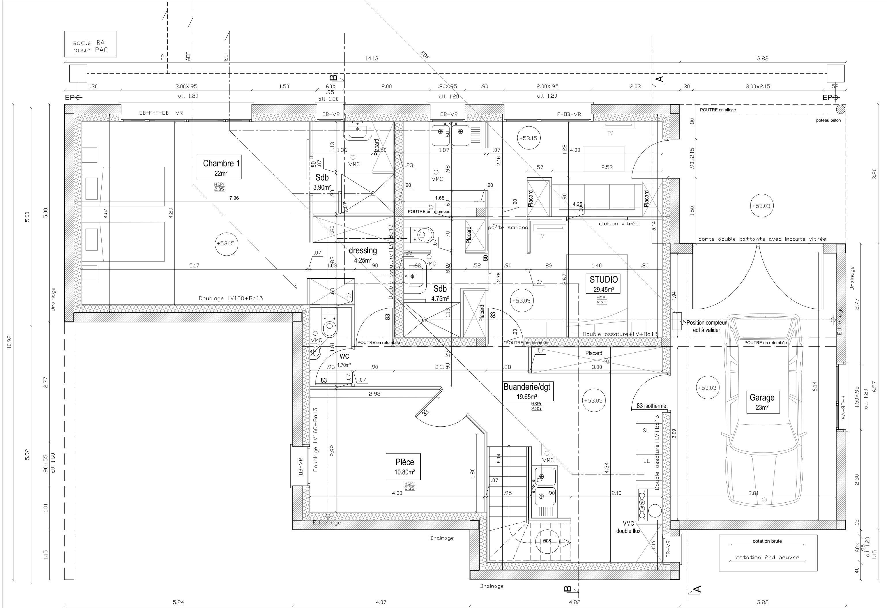
PLAN du Rez-de-Chausée Ech: 1/50
